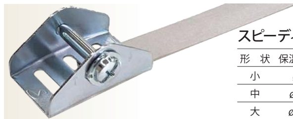
STEP 3 インパクトドライバーで締めます。
