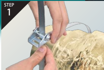
STEP 1 金具本体の穴にバンドを通します。
