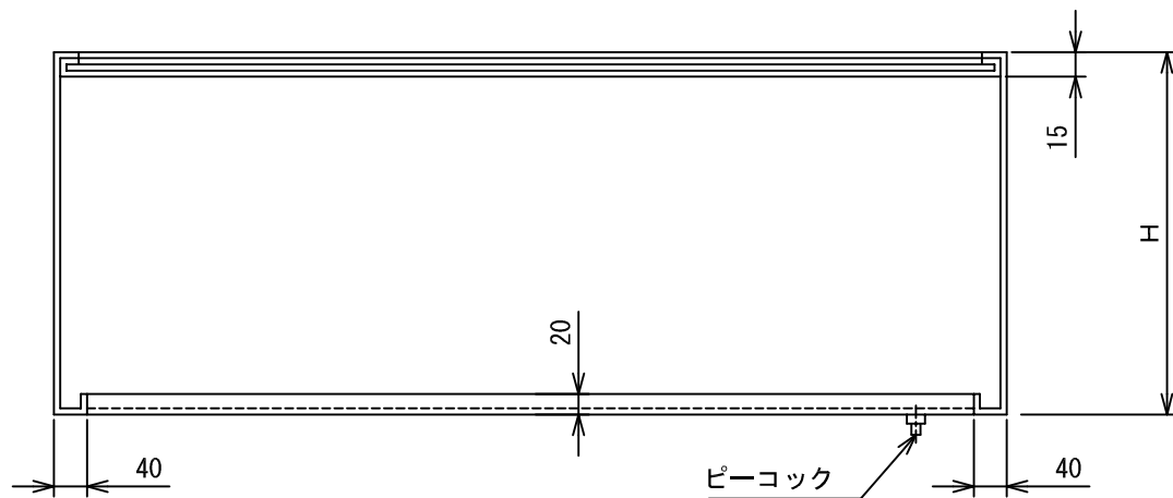
B-B断面図
