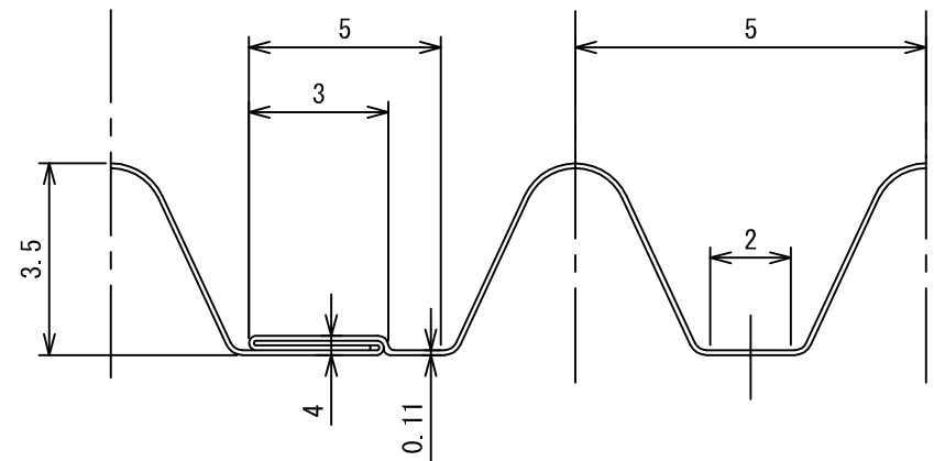
A部 詳細断面図
