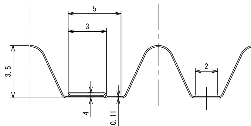
A部 詳細断面図
