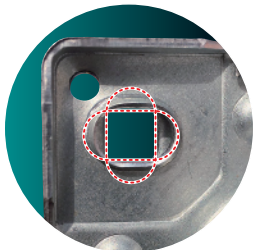
コーナーの長穴が十字に重なって根角ボルトを固定します。
